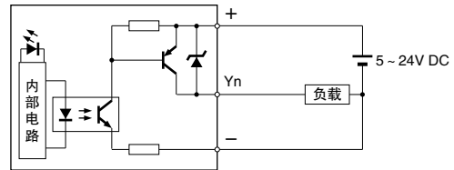
[ 输出电路·源型 ]
