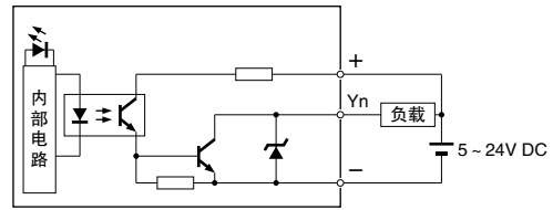
[ 输出电路·漏型 ]
