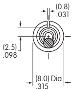
A1 .280" (7.1mm) 螺纹型有键槽
