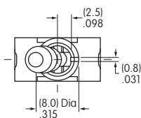
LL2 平滑有键槽
