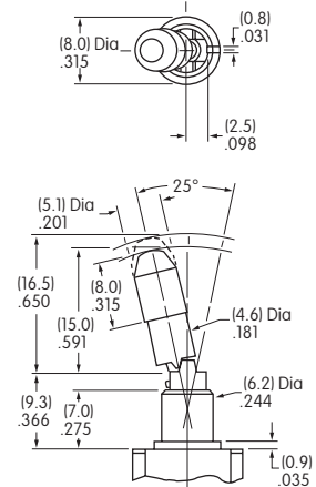
LL2 平滑型有键槽
