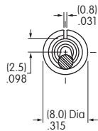
A2 .280" (7.1mm) 平滑有键槽
