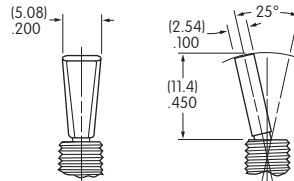
E .450" (11.4mm) 扁平
