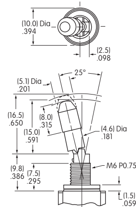
LL8 6mm/.295" (7.5mm) 防溅入螺纹D形衬套
