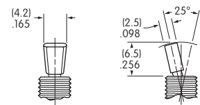
E2 .256" (6.5mm) 扁平
