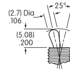
E2 .256" (6.5mm) 扁平
