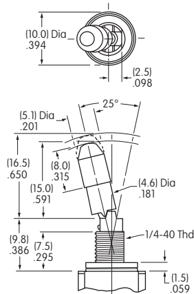
LL3 1/4-40 .295" (7.5mm) 防溅入螺纹D形衬套
