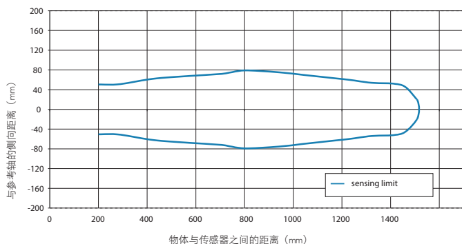
感应范围为200...1500mm的超声波传感器的典型声束 100x100mm标准目标物, 垂直于传感器的参考轴
