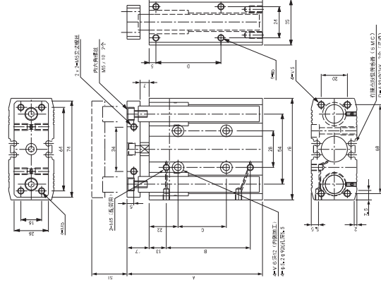
货号No. 060497 规格 06YL20-M-40 总行程：40mm 总重量：165g ※可安装限位传感器。
