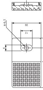
垫板·角型·黑·压入用
