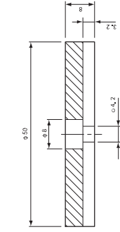
垫板·圆型·白 φ 50· 微型气缸用
