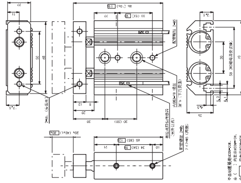
※由于是双杆构造，动作流畅。 货号No. 130708 规格 M20M-20W 总行程：20mm 总重量：112g ※可安装限位传感器。
