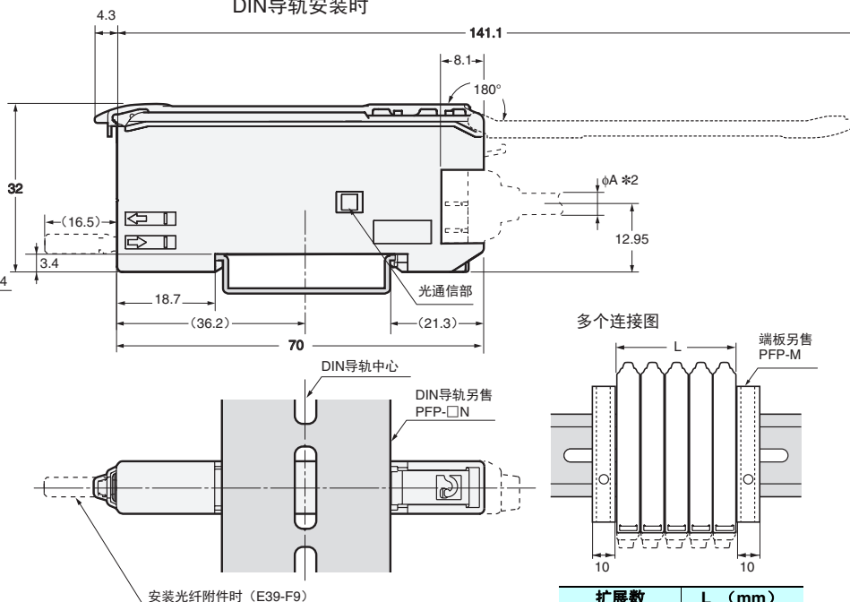
DIN导轨安装时
