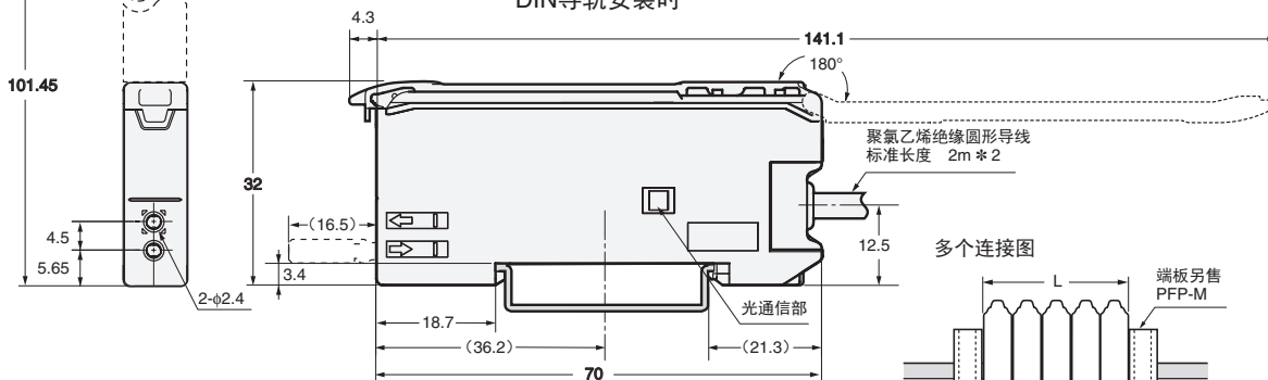
DIN导轨安装时
