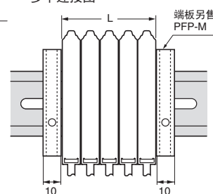
多个连接图
