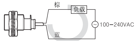
< 交流2线型 >
