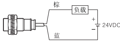
< 直流2线型 >
