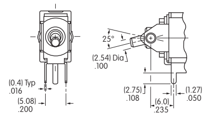
垂直PC端子安装
