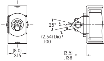
直型PC端子安装
