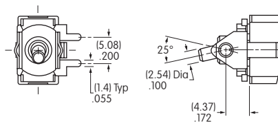
直角PC端子安装
