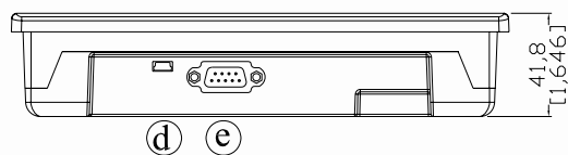
底视图
