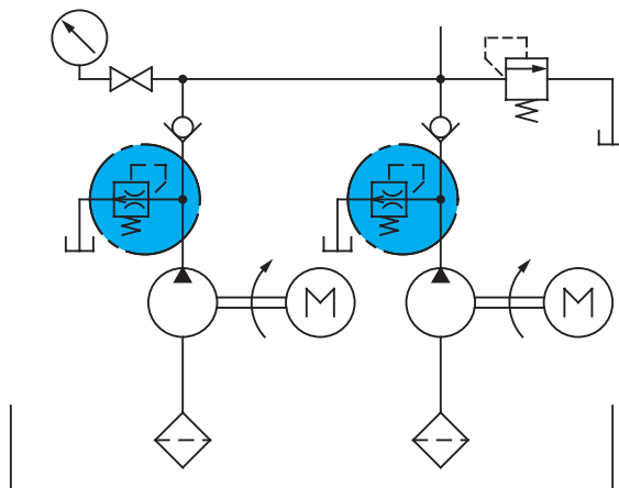
回路图B
